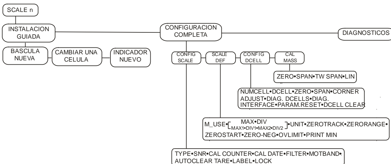
Figura 5.1.7 Menú báscula tipo digital
