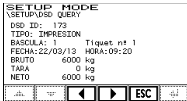
Figura 2.8.2.1.3 Consulta DSD: Visualización pesada
