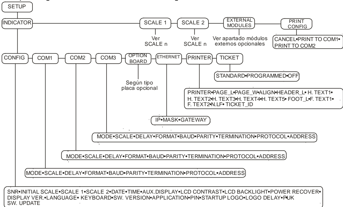
Figura 5.1.5 Esquema general del menú
