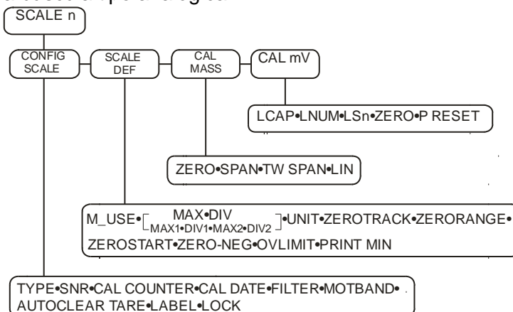
Figura 5.1.6 Menú báscula tipo analógica
